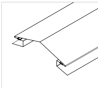
FAÎTIÈRE
